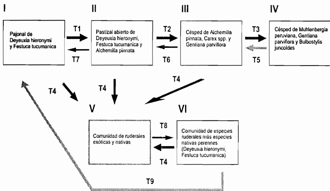
Figura 2, Esquema del modelo de estados y transiciones para los pastizales de altura de las Sierras de Córdoba, Argentina. Los números romanos indican diferentes estados; la caja gris del estado V indica inestabilidad; las flechas grises indican baja probabilidad de ocurrencia de la transición.
